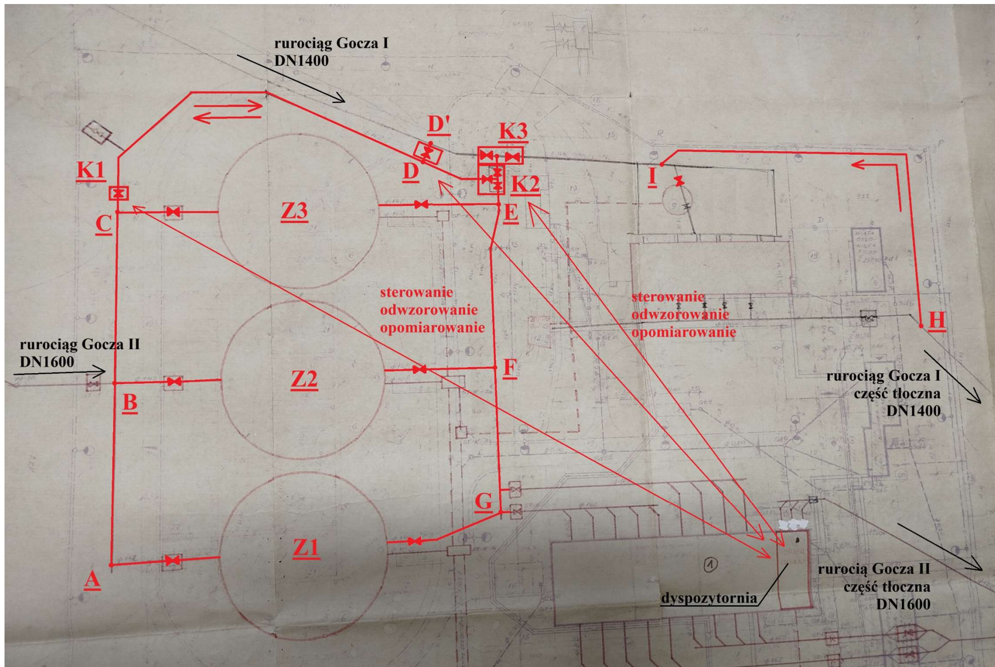
Załącznik nr 1 – schemat technologiczny Przepompowni Paprocany – zakres robót
